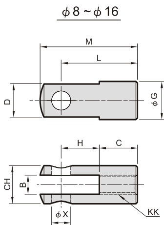
Y型、I型 接頭尺寸表：
