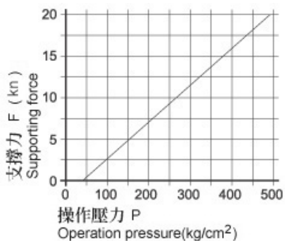
SP-25B 油压顶出型
