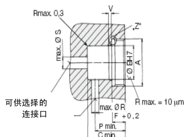
板式连接孔
