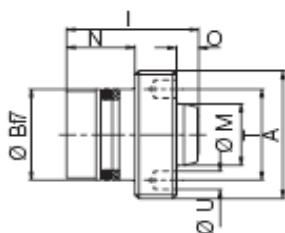
阳接口
