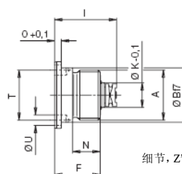
接口基座
