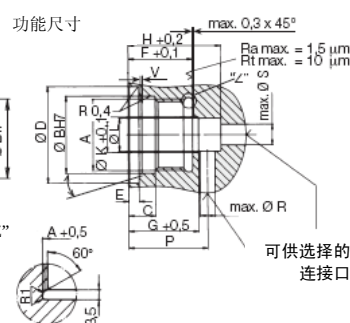
板式连接孔
